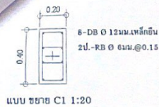
แบบ ขยาย C1 1:20
