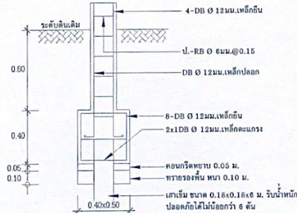
แบบ ขยาย F2 1:20
