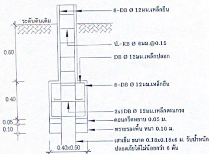
แบบ ขยาย F1 1:20
